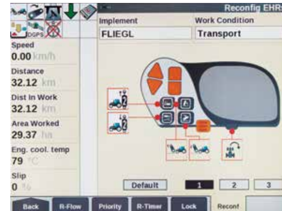
ISOBUS-funktioner kan konfigureras på befintliga reglage som Multicontroller, joystick och manöverspakar.
